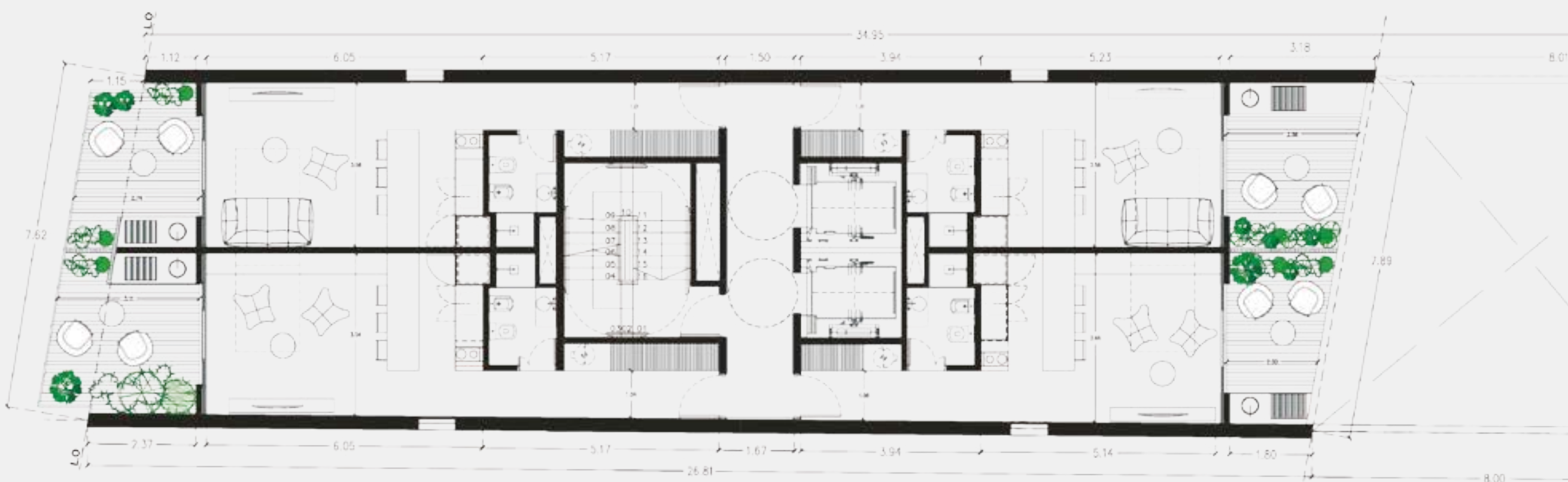
PLANTA TIPO 2° - 10°
